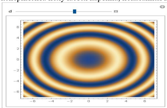
Рис. 2. Интерференционная картина, полученная по схеме, показанной на рис. 1.
