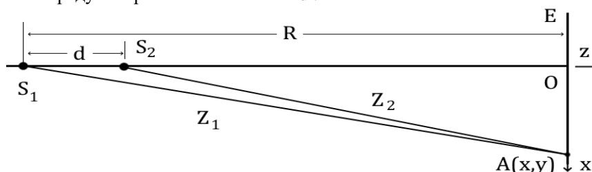
Рис. 1. Эквивалентная оптическая схема интерферометра Майкельсона.
