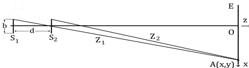
Рис. 4. Эквивалентная оптическая схема интерферометра Майкельсона для протяженных источников света
