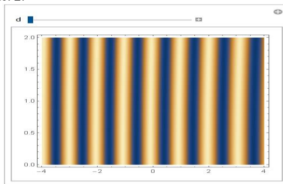
Рис. 3. Интерференционные полосы, формирующиеся при наклоне одного из зеркал на небольшой угол.
