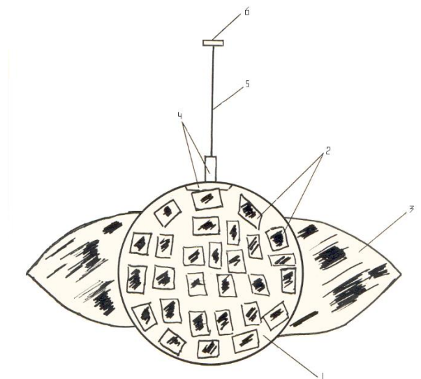
3-расм. Қушларни чўчитиб ҳайдаш учун қурилма.
