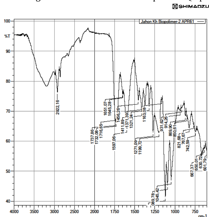
2-rasm. PL/mod-Sellyuloza/PVS kompozitining IQ-spektri
