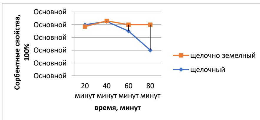
Рисунок 2. Сорбентные свойства глинистых порошков двух разных составов при активации при температуре 100°C.
