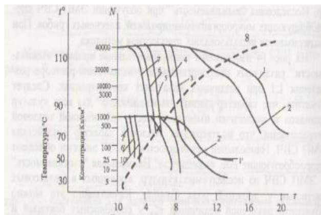
Расм-2. Турли бошланғич концентрациядаги мелассада микроорганизмлар «яшаш» эгри чизиги.
