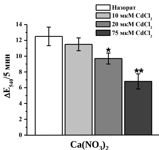
1-rasm. \text{Cd}^{2+} ionlarining mitoxondriya membranasi \text{Ca}^{2+} ionlari uchun passiv o'tkazuvchanligiga ta'siri * R < 0,05 , ** R < 0,01 , (n=5).
