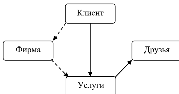
Рис.1. Идеальный NPS модель (Источник: Разработка авторов.)
