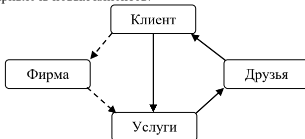
Рис.3. NPS модель с обратной связью (Источник: Разработка авторов.)
