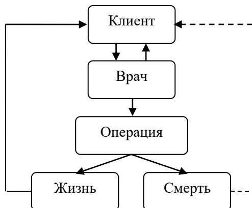
Рис.2. Пример NPS модели с обратной связью (Источник: Разработка авторов.)
