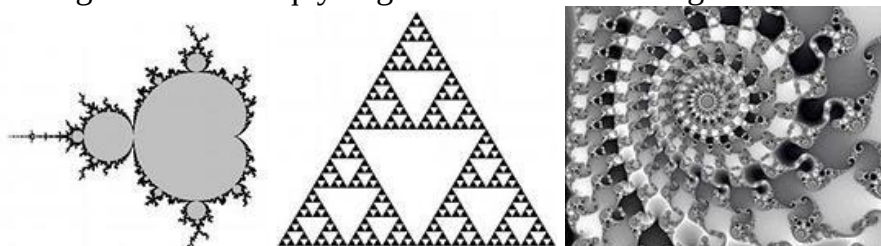
3-rasm. Fraktallarning ko‘rinishlari
