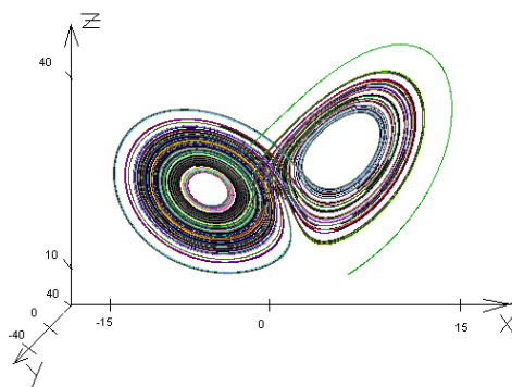
2-rasm. Attraktorning umumiy ko‘rinishi
